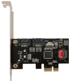
Adaptador PCI-Express 2 x SATA internos - ECO. PCI-Express Adapter, 2 internal SATA Ports - ECO.
