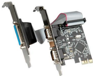
PCI-Express 2 x Serie RS232 Sub-D9 + 1 x EPP/ECP - ECO. PCI-Express Ad., 2 x Ser. RS232 D-Sub 9 + 1 x EPP/ECP - ECO.
